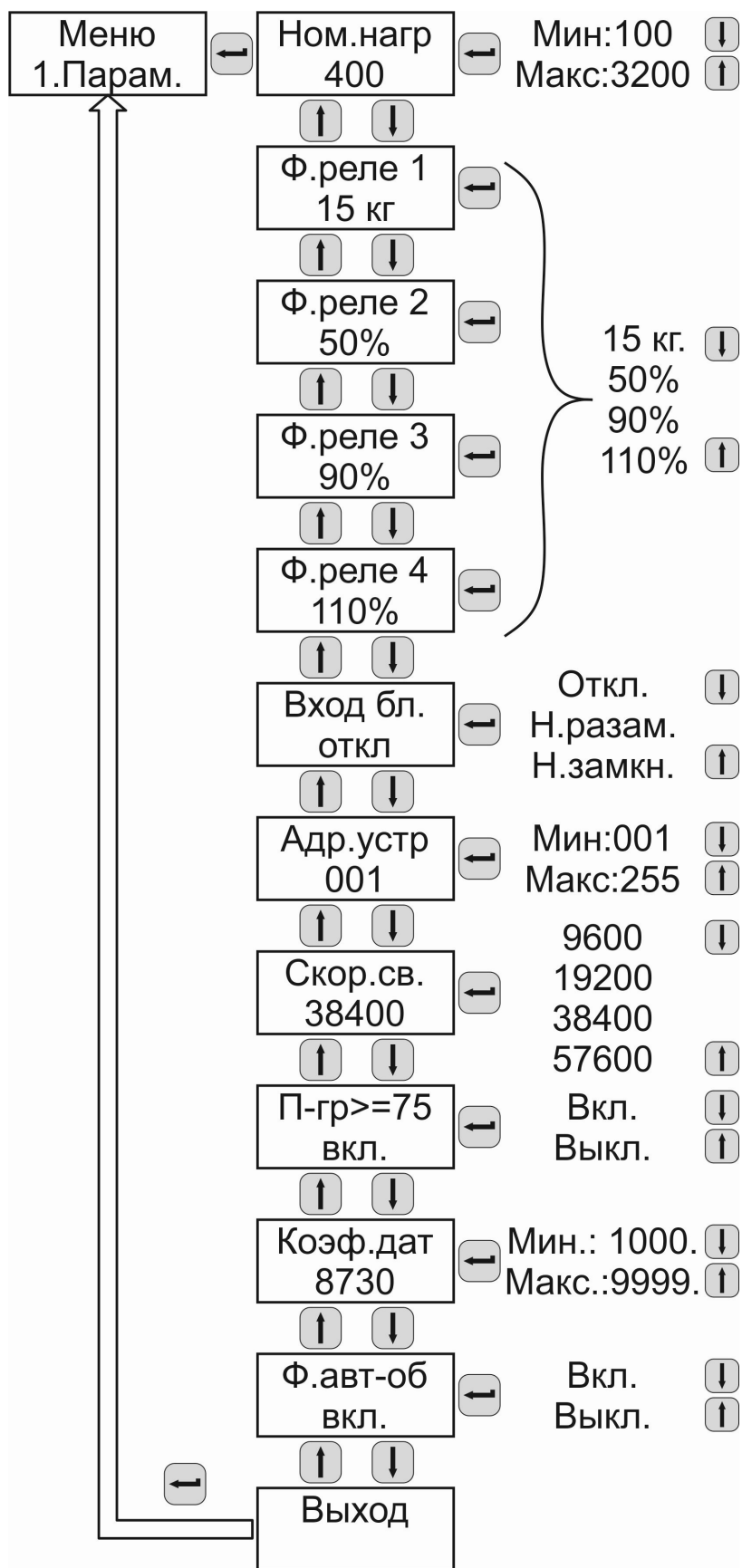
Рисунок 7 – структура меню параметров.
