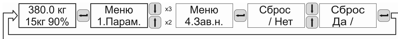
Рисунок 10 – Структура функции сброс к заводским настройкам.
