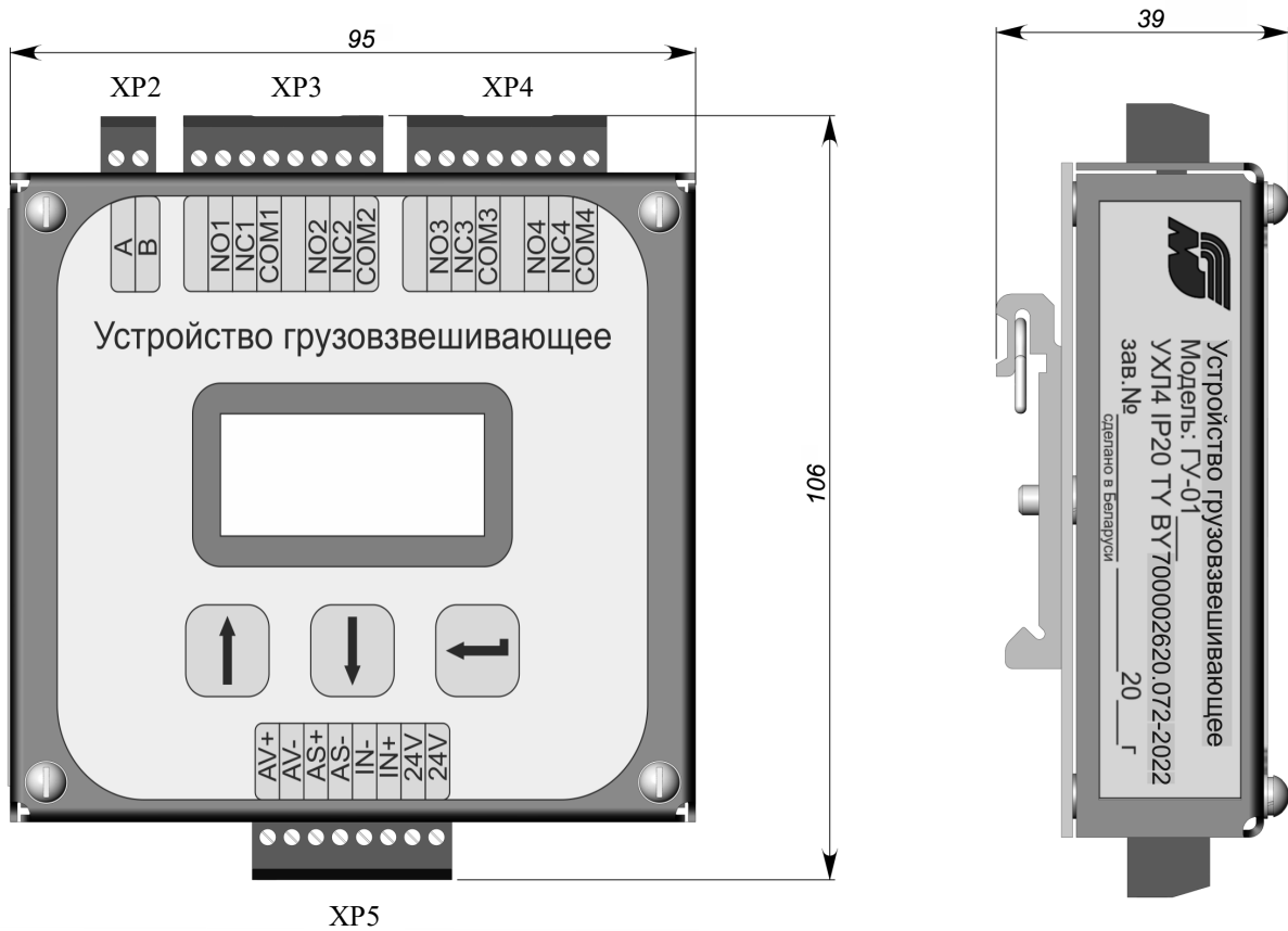
Рисунок 1 – Габаритные размеры блока
