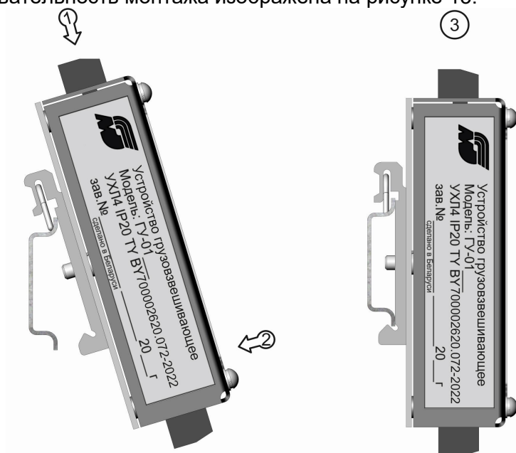
Рисунок 13 – Последовательность монтажа блока контроля на DIN-рейку.
